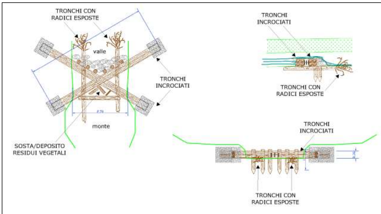
Figura 37 - Schema progettuale di massima dell'intervento di costruzione di strutture trasversali atte ad aumentare la capacità di sedimentazione e rialzare il livello dell'alveo Immagine: Consorzio di Bonifica dell'Emilia Centrale (RE).
