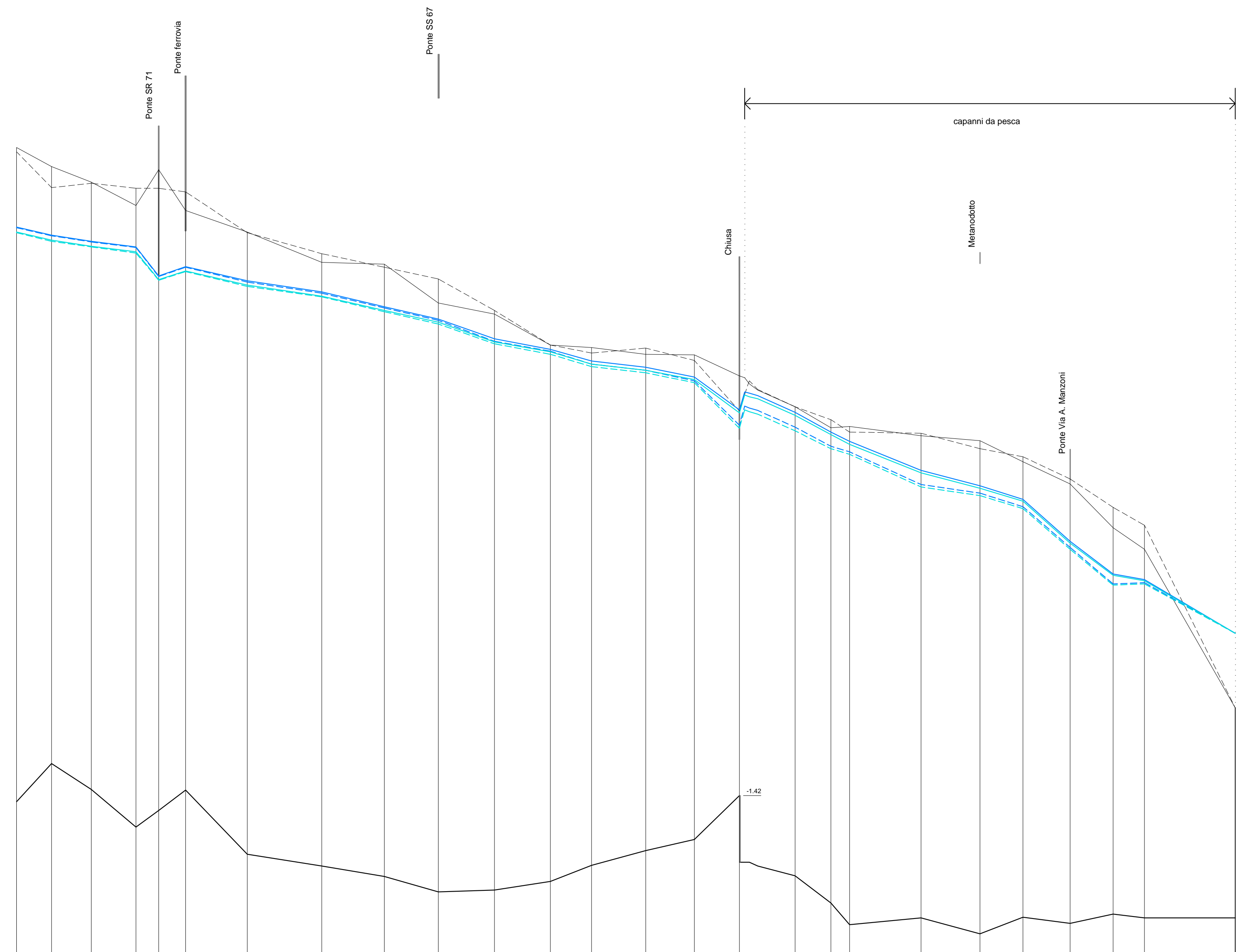
TAV. 8 - Profili del pelo libero dei Fiumi Uniti per gli eventi di piena di tempo di ritorno T=100 e 200 anni, nelle condizioni di esondazioni libere, in assenza ed in presenza di capanni da pesca
