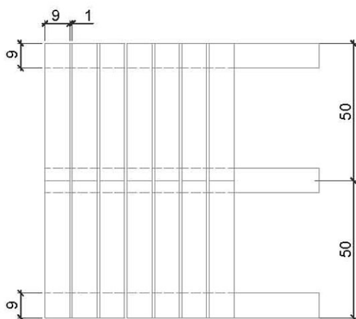
POSA CON FUGHE – ESEMPIO B2 (quote in cm)
