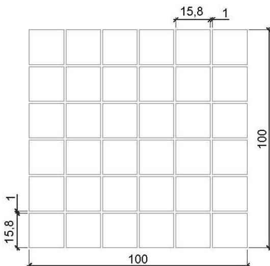
POSA CON FUGHE – ESEMPIO B1 (quote in cm)
